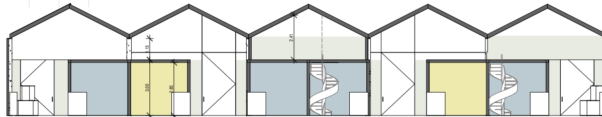
SEZIONE TIPOLOGICA
